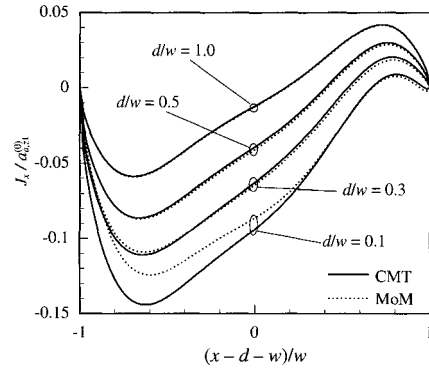
(d) J_x for the asymmetric mode.
