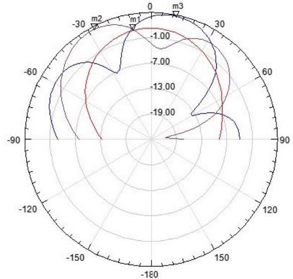
Elevation Pattern Gain Display (dB) m1 = Freq - '4.37 GHz' Phi = '9 deg' m2 = Freq - '7.74 GHz' Phi = '9 deg' m3 = Freq - '10.67 GHz' Phi = '9 deg'
