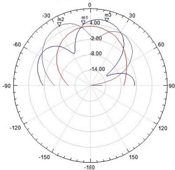
m1 = Freq - '4.37 GHz' Phi = '9 deg' Mag - 4.08 m2 = Freq - '7.74 GHz' Phi = '9 deg' Mag - 6.19 m3 = Freq - '10.67 GHz' Phi = '9 deg' Mag - 5.89
