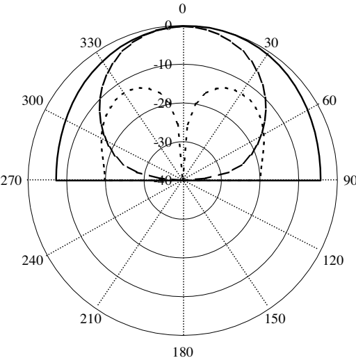
(d) 9 GHz
