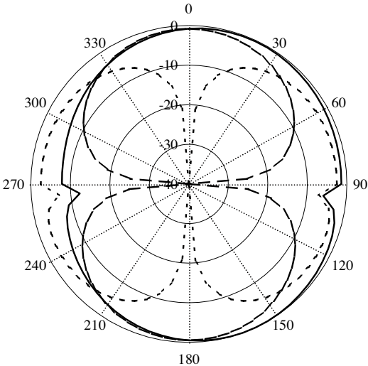
(b) 10 GHz
