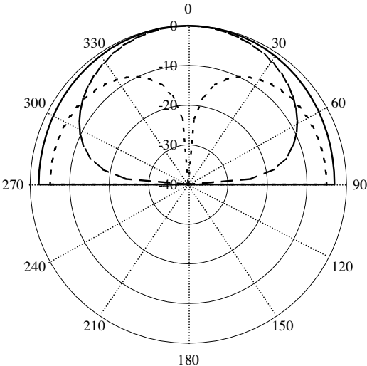
(b) 5 GHz
