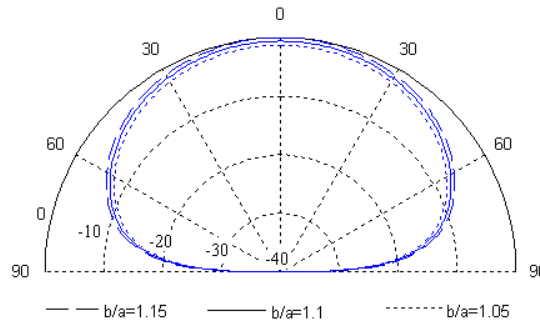
(a) H -plane patterns.
