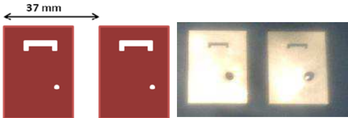
Figure 4. The 1 \times 2 linear array antenna.
