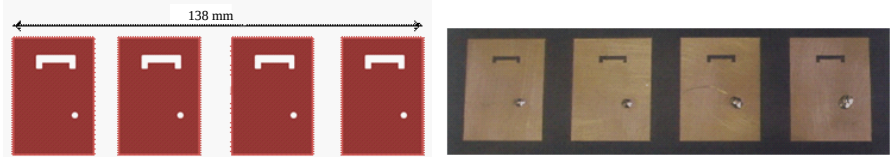
Figure 7. The 1 \times 4 linear array antenna.
