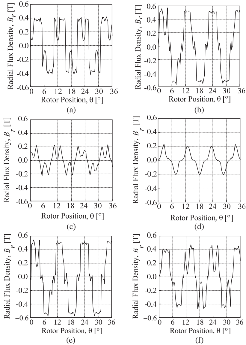
Figure 5. Radial flux density of DSPM motor. (a) DSPM-ST. (b) DSPM-AP. (c) DSPM-DP. (d) DSPM-IP. (e) DSPM-CR. (f) DSPM-SR.
