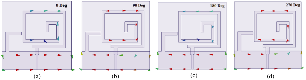
Figure 4. Surface current distribution at 2.45 GHz. (a) 0^\circ . (b) 90^\circ . (c) 180^\circ . (d) 270^\circ .
