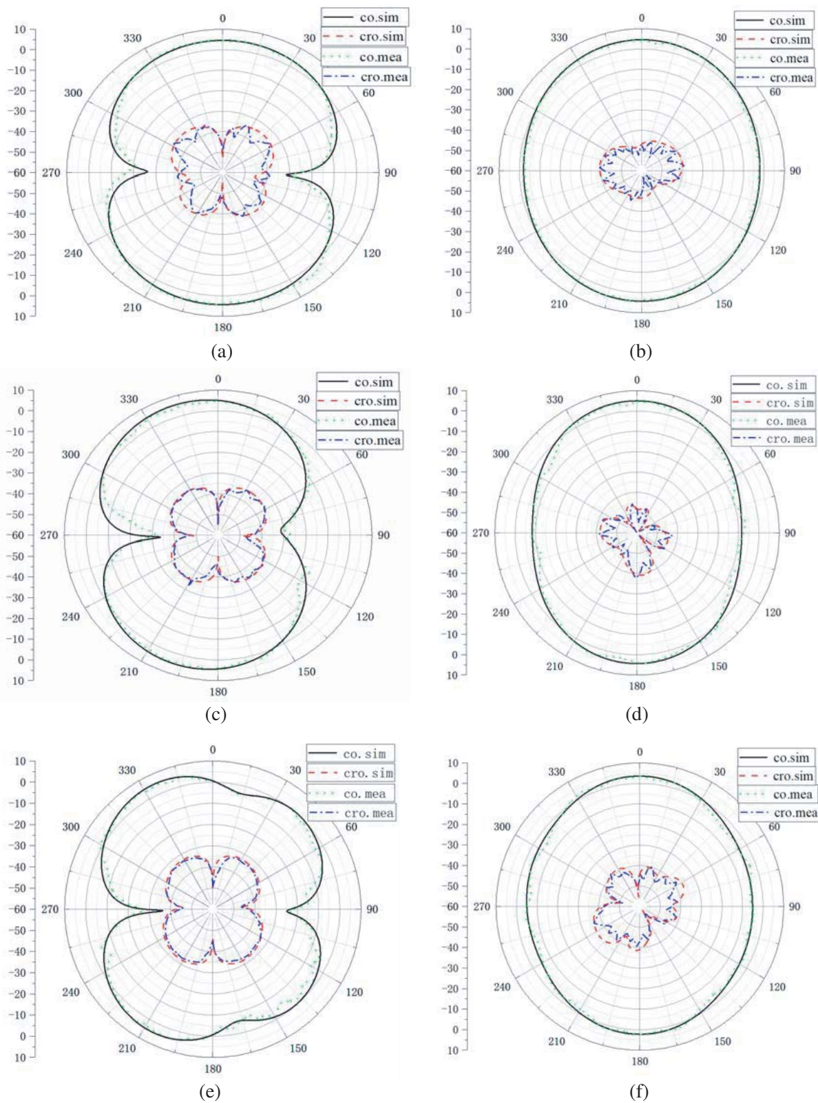
Figure 9. Radiation pattern of the E -plane and the H -plane. (a) E -plane at 4 GHz. (b) H -plane at 4 GHz. (c) E -plane at 6 GHz. (d) H -plane at 6 GHz. (e) E -plane at 9 GHz. (f) H -plane at 9 GHz.
