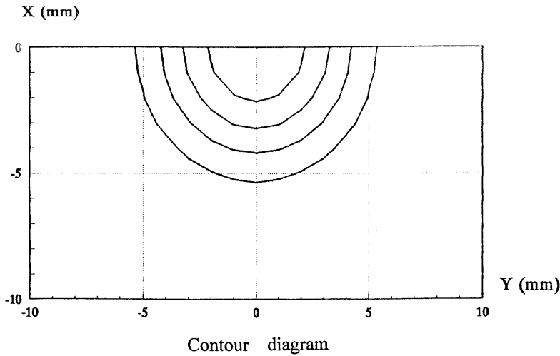
(a) Oblique angle \theta_0 = 0^\circ .
